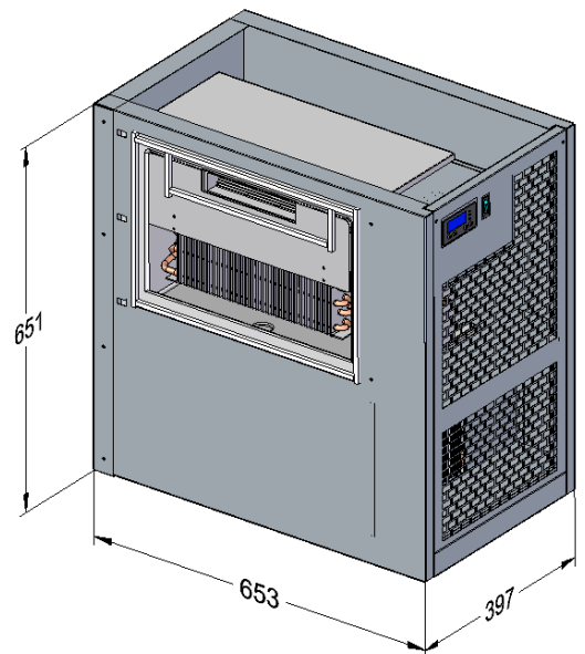
Abbildung KSS405 mit Maschinenfach für Kühltisch:
